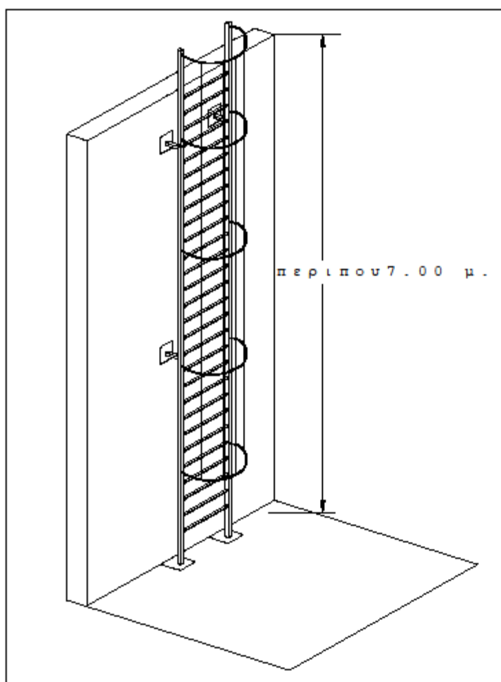
στηρίξη τοίχου
