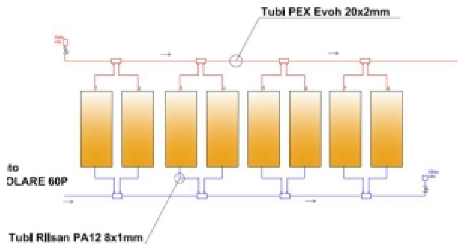
Ρακόρ για τη σύνδεση των σωλήνων PA12 8X1mm με την υδραυλική υποδοχή στην οπίσθια πλευρά των PV/T πλαίσιων
