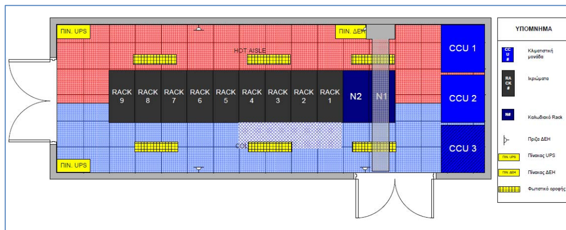
Σχήμα 1. Χωροθέτηση ηλεκτρομηχανολογικών υποδομών datacenter
