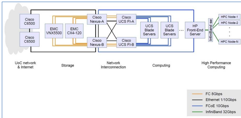
Σχήμα 2. Αρχιτεκτονική διάταξη υφιστάμενων υποδομών datacenter
