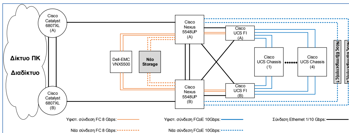
Σχήμα 3: Αρχιτεκτονική διάταξη συνδεσμολογία DC με τις προσθήκες του νέου storage και των δυο νέων εξυπηρετητών. Με γκρι χρώμα παρουσιάζονται τα υπό προμήθεια είδη.
