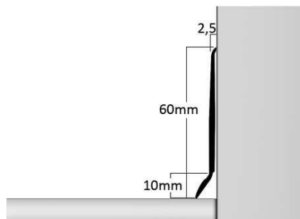
Εικόνα 34 Διαστάσεις Σοβατεπί
